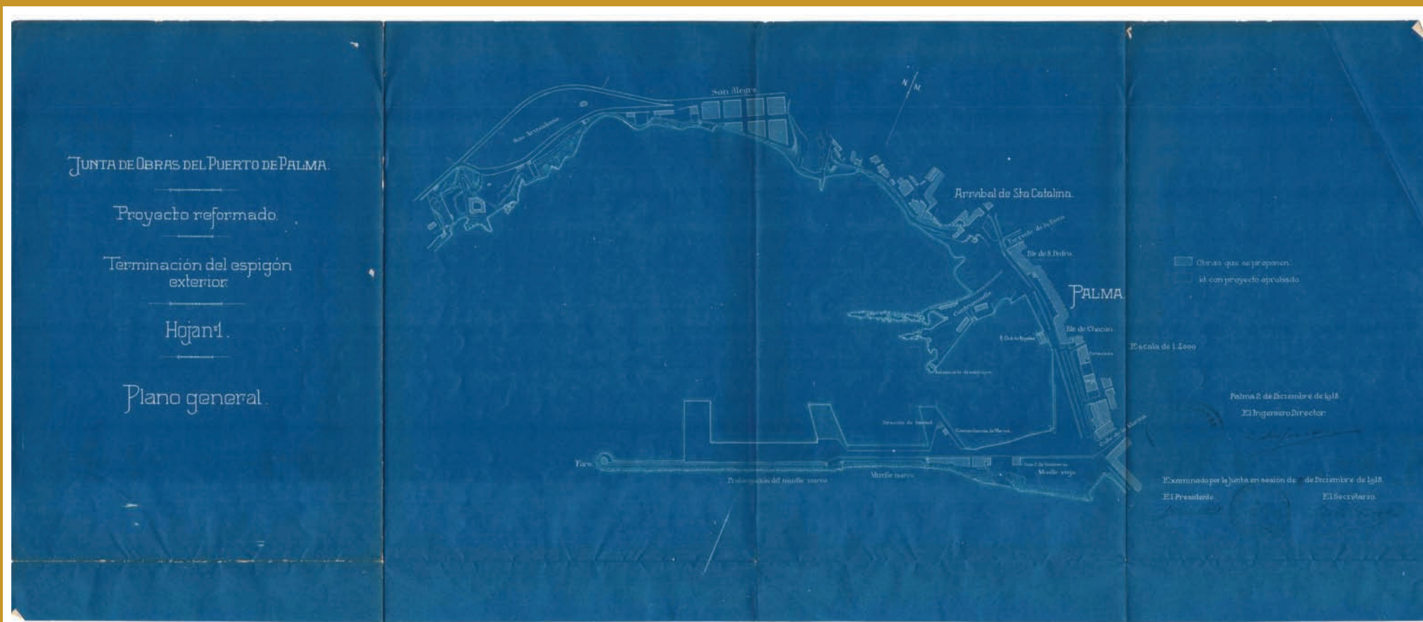
Fig. 21. Planta general de tercer projecte reformat del projecte Ensanche del Muelle Viejo , distribució de les zones de serveis i urbanització de terrenes sobrants, redactat per Pedro Carau l'any 1918.
