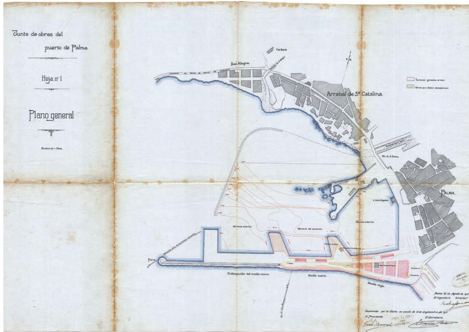
Fig. 16. Vista general del projecte Ensanche del Muelle Viejo , distribució de les zones de servicis i urbanizació de terrenes sobrants, redactat per Pedro Garau l'any 1911.
