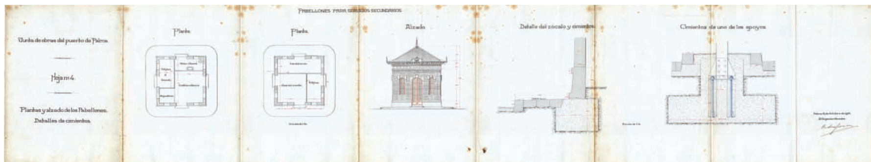
Fig. 25. Detall dels pavellons per a serveis secundaris del projecte Instalación de depósitos, grúas eléctricas de 3.000 kg y pabellones para servicios secundarios , redactat per Pedro Garau l'any 1913.
