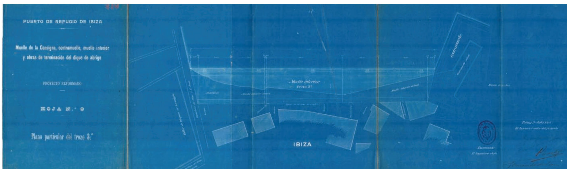
Fig. 34. Pla del Moll Interior del projecte Reformat del Muelle de la Consigna, Contramuelle, Muelle Interior y obras de terminación del dique de abrigo, redactat per Pedro Garau l'any 1904.
