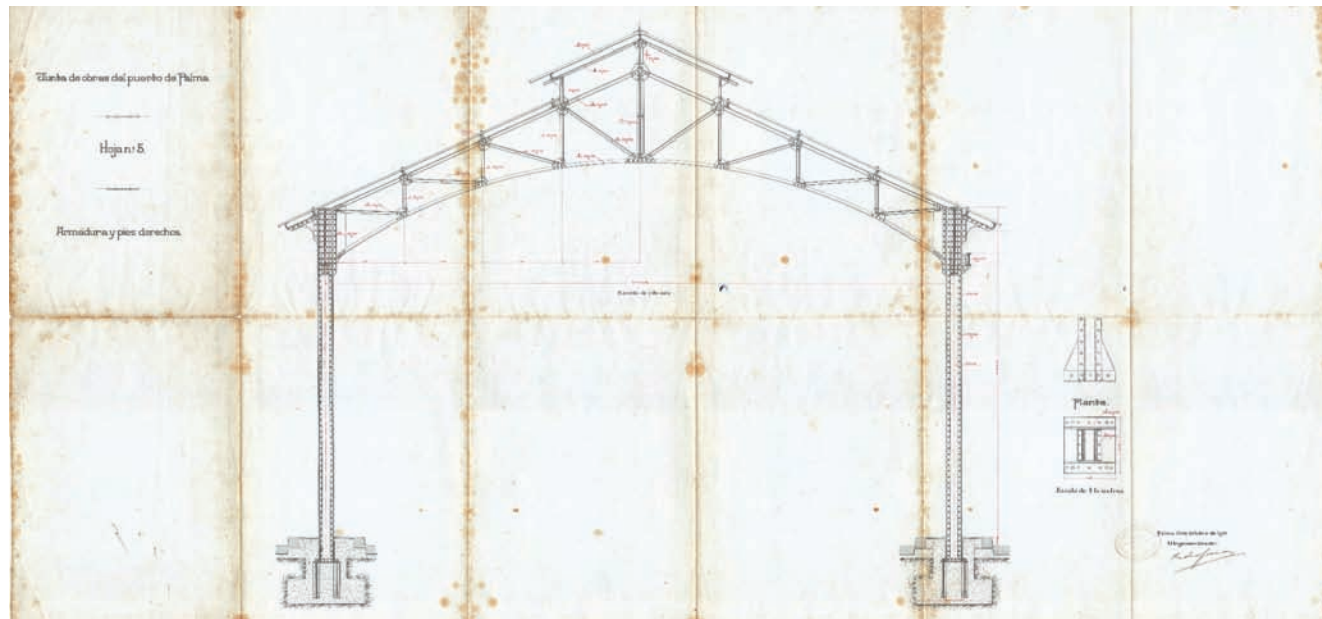
Fig. 24. Detall dels pavellons per als serveis secundaris del projecte Instalación de depósitos, grúas eléctricas de 3.000 kg y pabellones para servicios secundarios , redactat per Pedro Garau l'any 1913.
