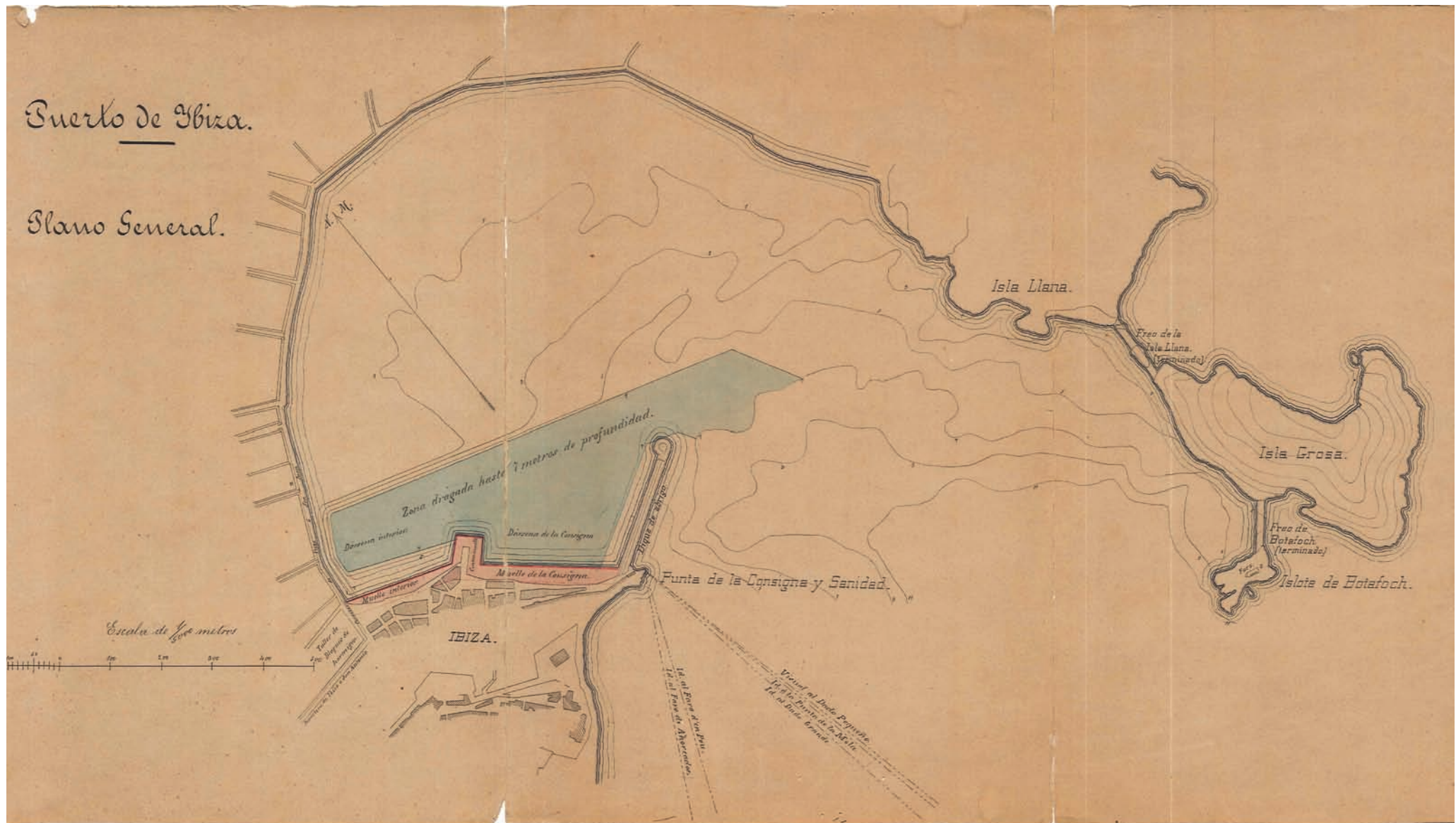
Fig. 30. Planta de conjunt del Proyecto reformado del Muelle Consigna, contramuelle y Muelle Interior, redactat per Pedro Garau l'any 1897.
