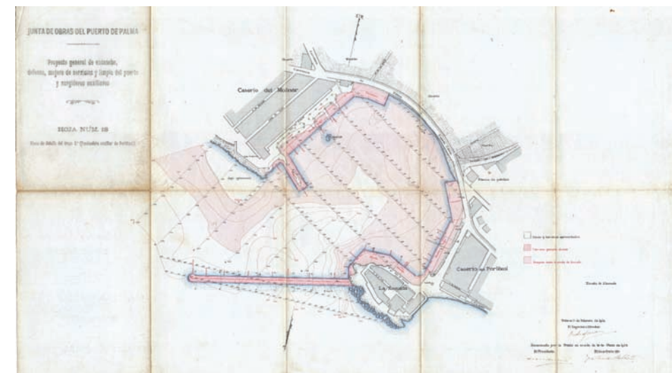
Fig. 9. Millora de la dàrsena del Portixol en el Proyecto general de ensanche, defensa, mejora de servicios y limpia del puerto de Palma y surgideros auxiliares, redactat per Pedro Garau Cañellas l'any 1913.
