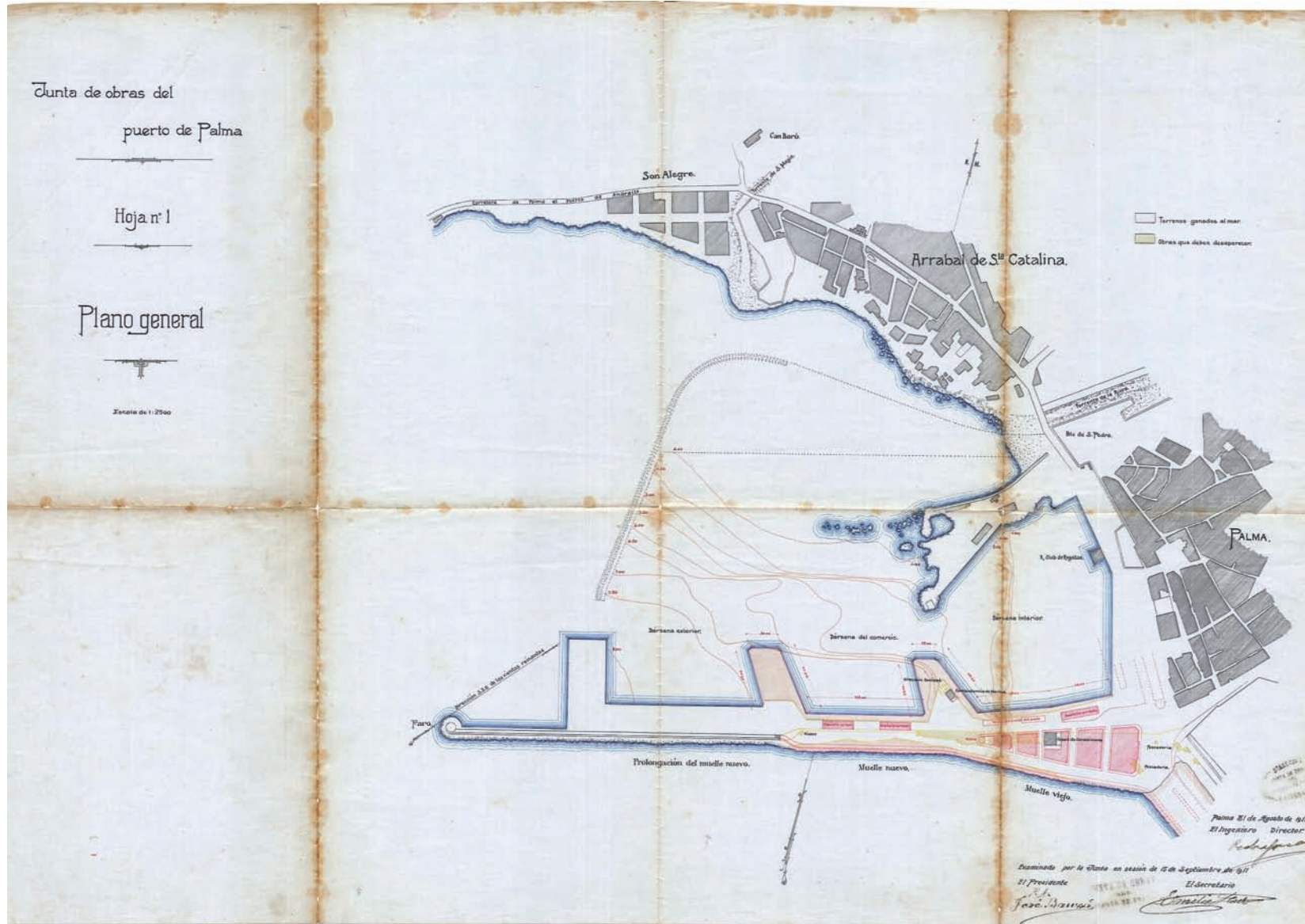
Vista general del projecte Ensanche del Muelle Viejo , distribució de les zones de serveis i urbanització de terrenys sobrants, redactat per Pedro Garau l'any 1911.
