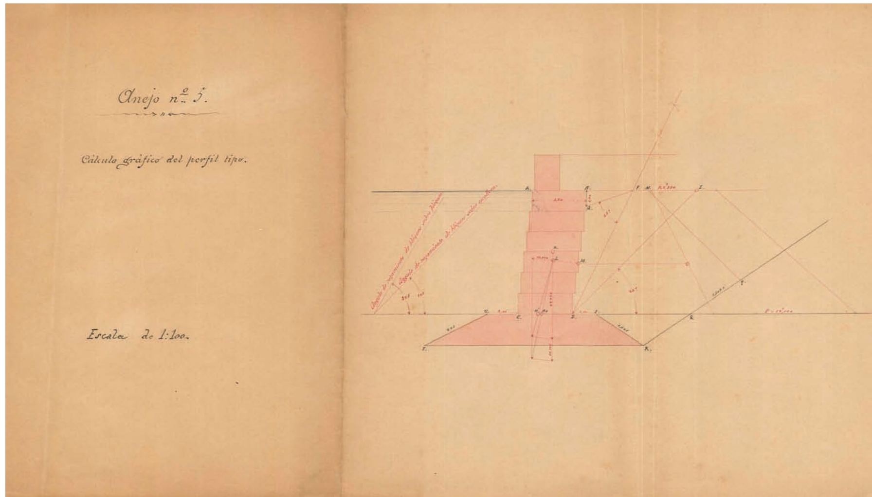
Fig. 31. Detalls del càlcul del Proyecto reformado del Muelle Consigna, Contramuelle y Muelle Interior , redactat per Pedro Garau l'any 1897.
