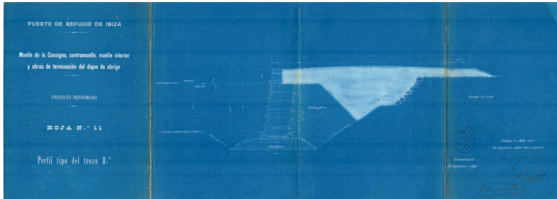
Fig. 35. Secció dels molls en el projecte Reformado del Muelle de la Consigna, Contramuelle, Muelle Interior y obras de terminación del dique de abrigo, redactat per Pedro Carau l'any 1904.
