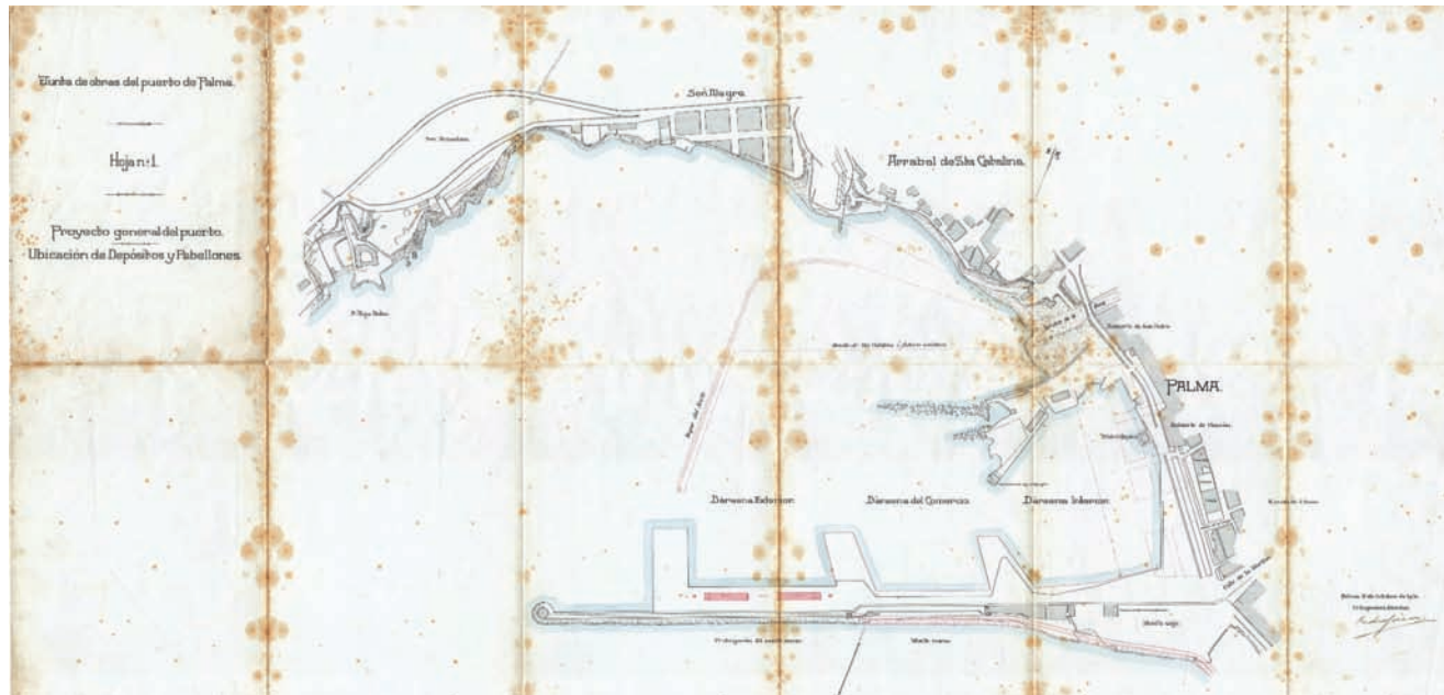
Fig. 22. Ubicació de dipòsits i pavellons del projecte Instalación de depósitos, grúas eléctricas de 3.000 kj y pabellones para servicios secundarios , redactat per Pedro Garau l'any 1913.
