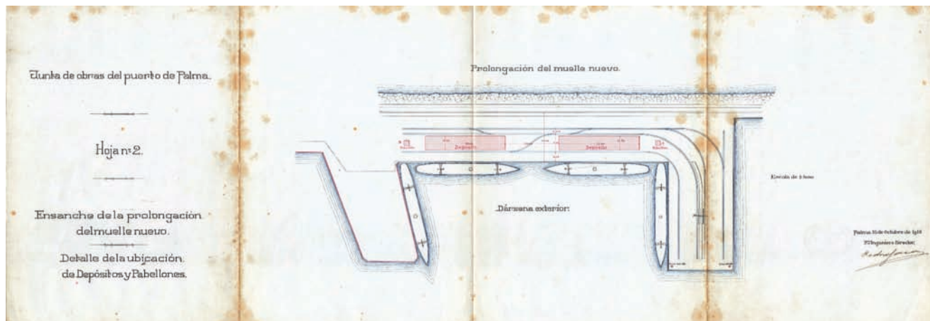
Fig. 23. Detall de la ubicació de dipòsits i pavellons del projecte Instalación de depósitos, grúas eléctricas de 3.000 kj y pabellones para servicios secundarios , redactat per Pedro Garau l'any 1913.
